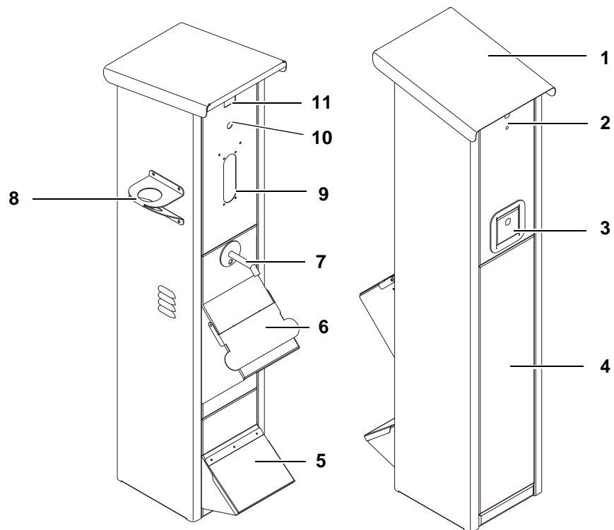
Abb. 2-2 Übersicht Entsorgungssäule
