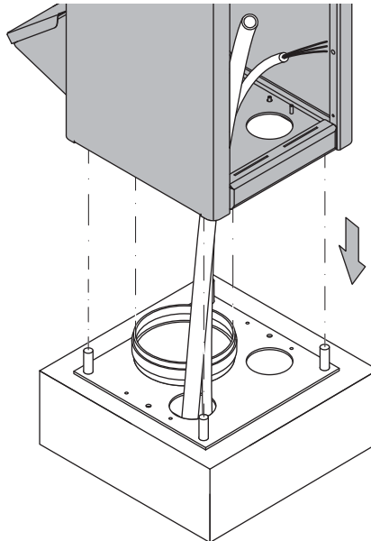
Abb. 5-8 Entsorgungssäule auf Abflussrohr aufsetzen
