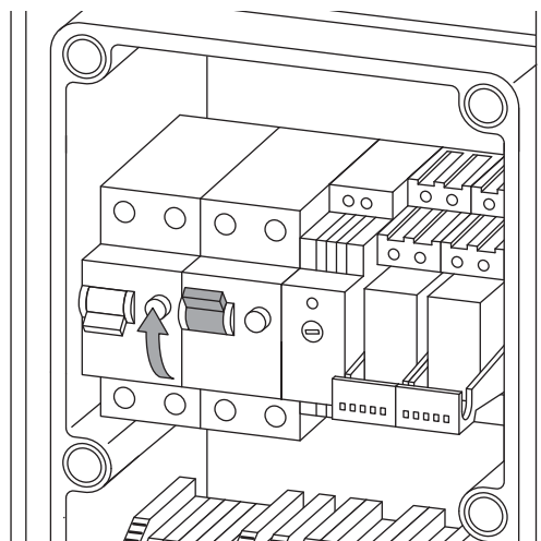
Abb. 6-12 Sicherung Heizung EIN
