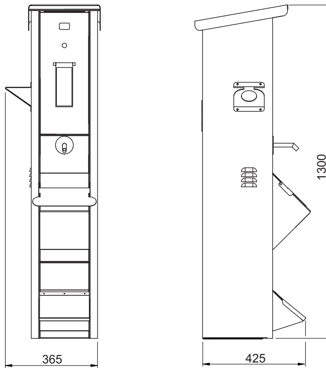
Abb. 2-1 Abmessungen
