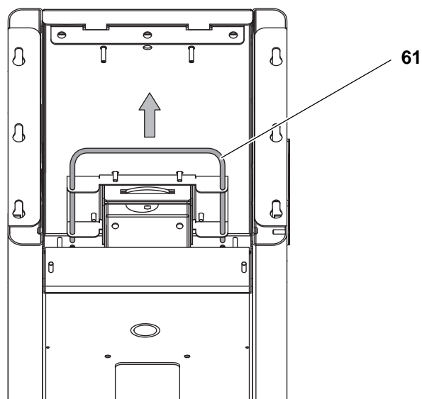
Abb. 6-3 Entriegelungshebel für die hintere Abdeckung
