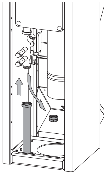
Abb. 5-10 Wasserleitung an Haupthahn anschließen
