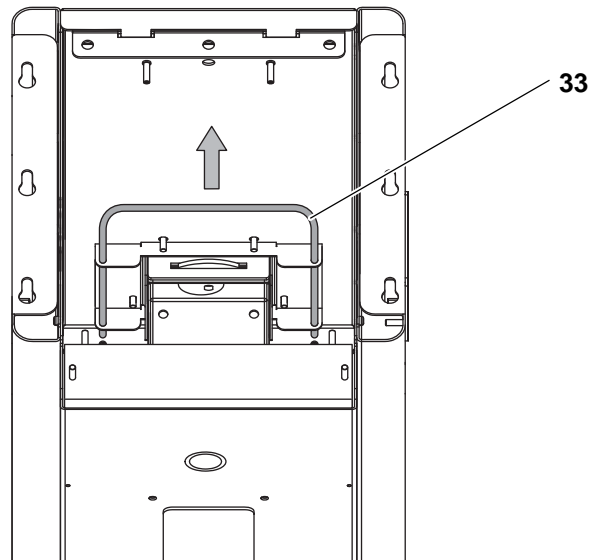
Abb. 6-26 Entriegelungshebel für die hintere Abdeckung
