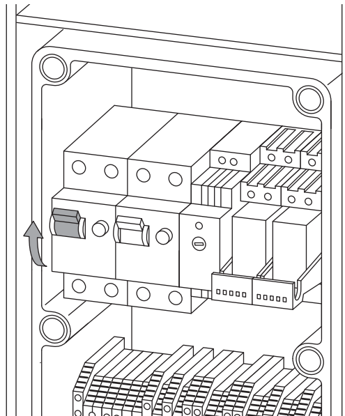
Abb. 6-6 Sicherung Steuerung EIN
