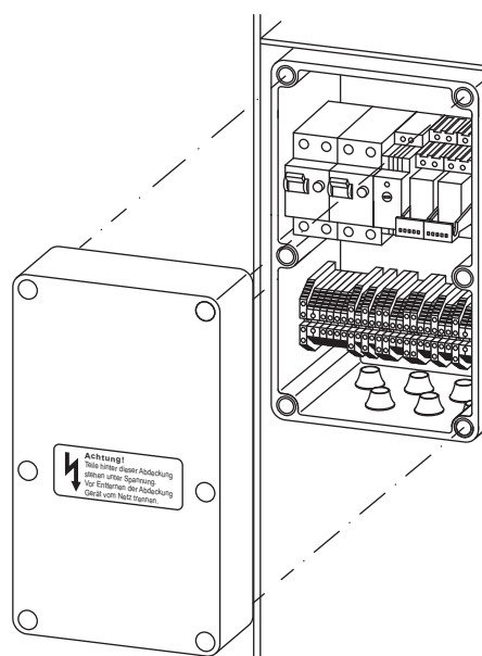
Abb. 3-3 Warningschild Isobox-Schaltkasten
